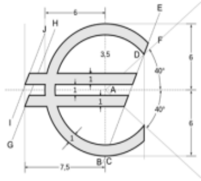
Dibujo técnico del símbolo monetario del euro.
